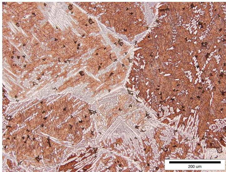
Slika 36. Optičke mikrografije uzorka legure Cu - 8,56 Al - 10,56 Mn - 0,5 Zr nakon kovanja, uzdužni presjek
