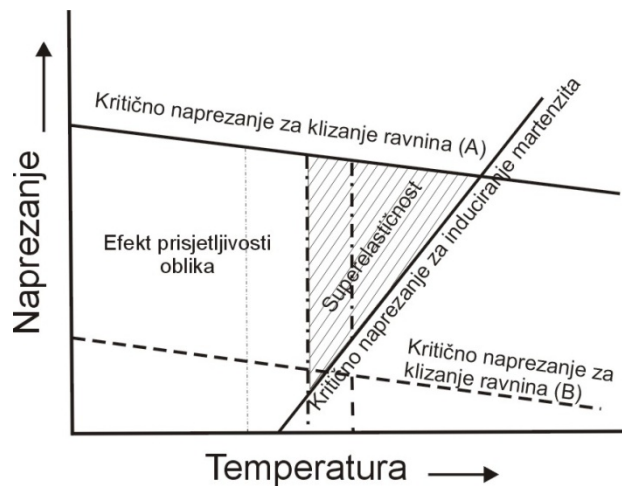
Slika 7. Shematski prikaz područja efekta prisjetljivosti oblika i superelastičnosti u ovisnosti o temperaturi i naprežanju [3]
