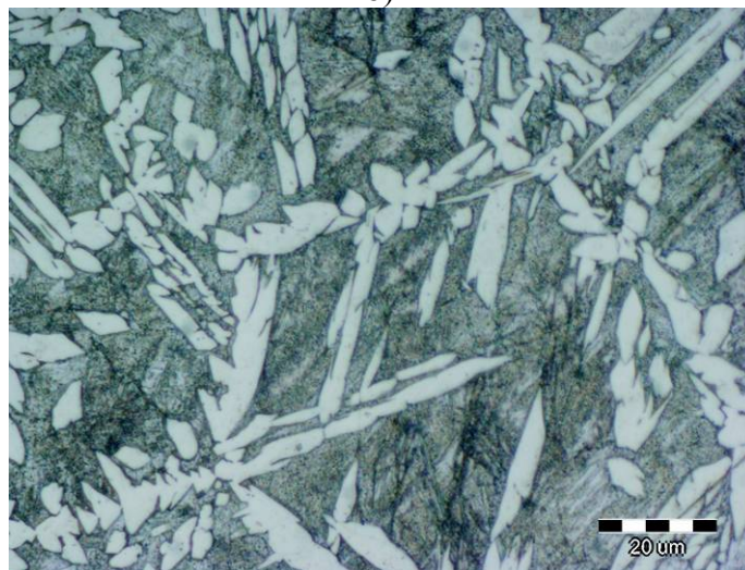
Slika 21. Optičke mikrografije CuAlMn brzo skrutnute trake pri povećanjima 100x (a), 500x (b) i 1000x (c), pozicija 1
