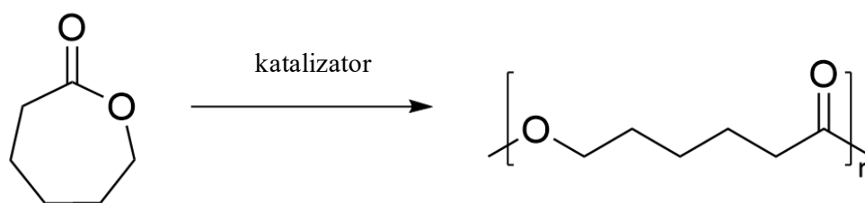
Slika 14. Sinteza polikaprolaktona [38]
