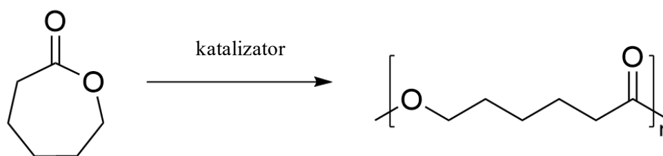
Slika 14. Sinteza polikaprolaktona [38]
