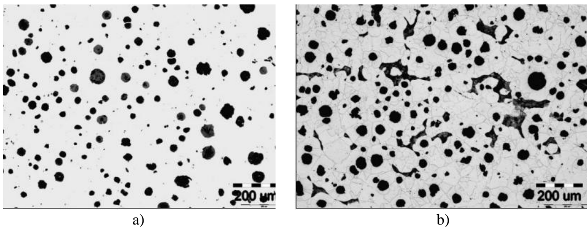
Slika 4. Mikrostruktura feritno – perlitnog nodularnog lijeva [8]: a) nenagrizenog stanja, b) nagrizenog stanja, nital
