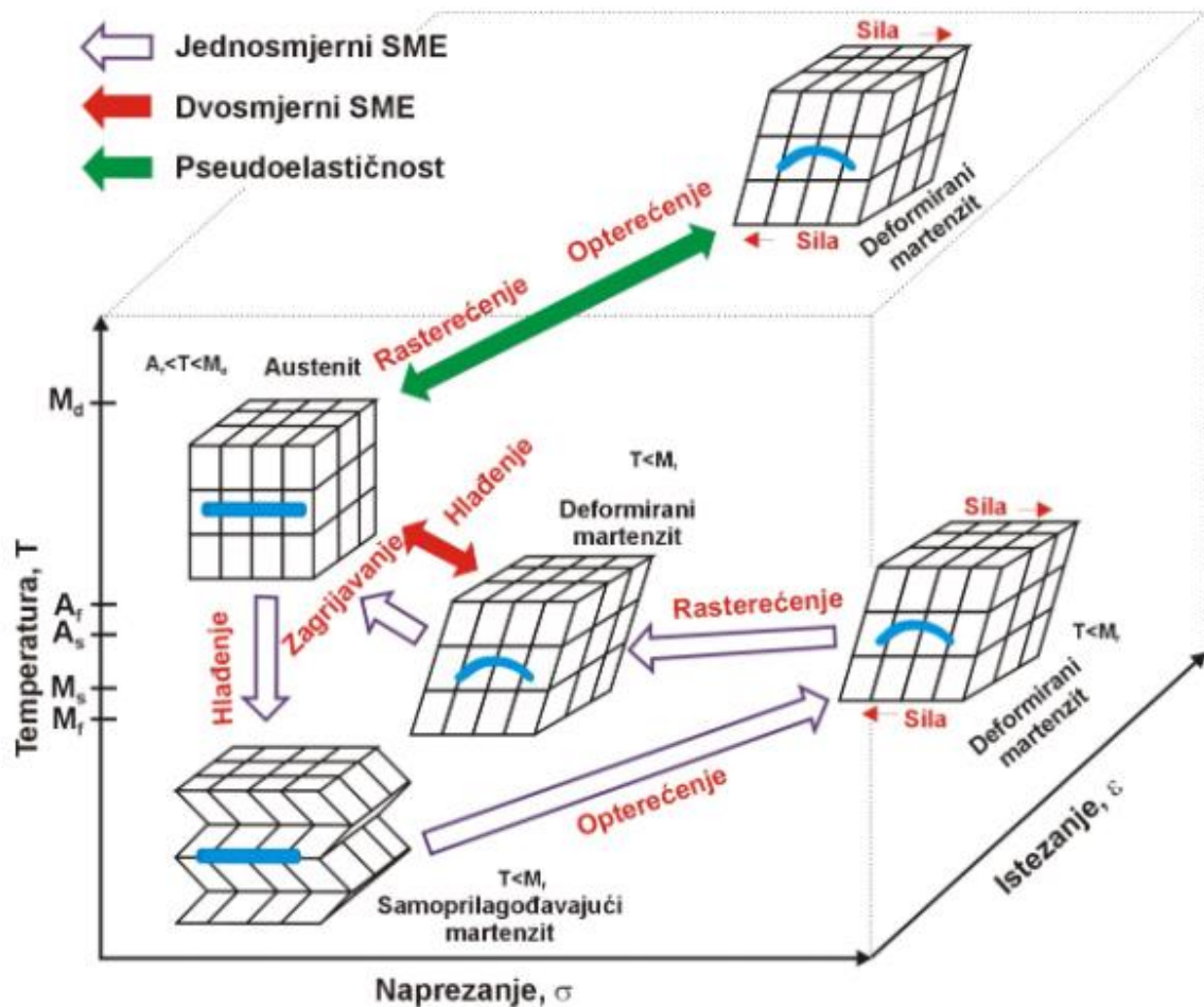
Slika 9. Kristalne strukture i faze legura s prisjetljivosti oblika (T – samoprilagođavajući martenziti, DT – naprezanjem inducirani martenziti) [3]
