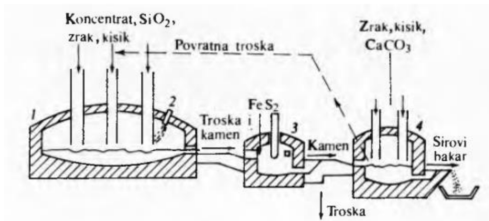
Slika 5. Kontinuirani postupak proizvodnje bakra, Mitsubishi postupak [8] 1. Peć za taljenje, 2. Gorionik, 3. Električna peć za preradbu troske, 4. Konvertor.
