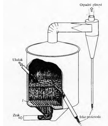
Slika 2. Peć za prženje u fluidizacijskom sloju [8]
