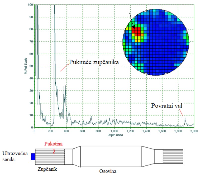
Slika 11. Pukotina na vratilu uočena ultrazvučnim ispitivanjem [26]
