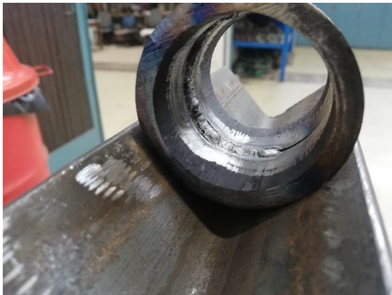
Slika 10. Fotografija korijena zavara a) i konačnog zavarenog spoja b)
