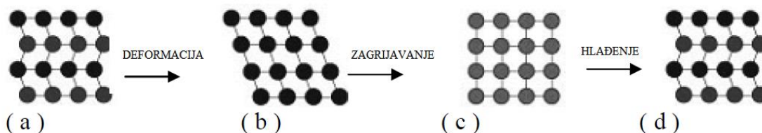
Slika 3. Prikaz jednosmjernog efekta prisjetljivosti oblika [10]
