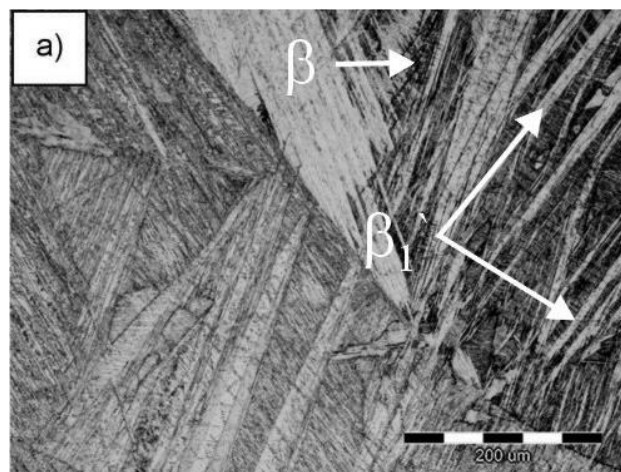
Slika 14. Primjer OM mikrofotografije martenzitne strukture u Cu-Al-Mn leguri [24]
