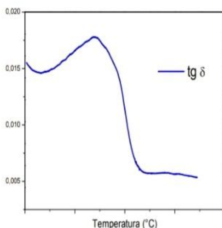
Slika 23. a) Promjena modula pohrane ( E' ) i modula gubitka ( E'' ) s temperaturom za leguru Cu-Al-Mn, b) promjena kuta gubitka ( \text{tg } \delta ) [28]
