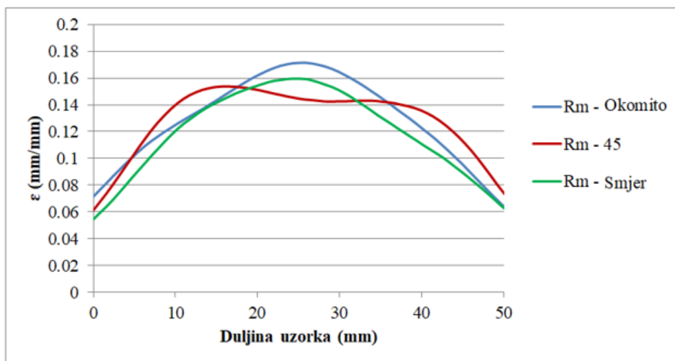
Slika 68. Linijska analiza promjene deformacije duž ispitnog uzorka za točke R_m
