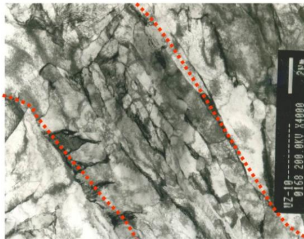
Slika 4. Prikaz rekristalizacije u deformiranom zrnima [1]
