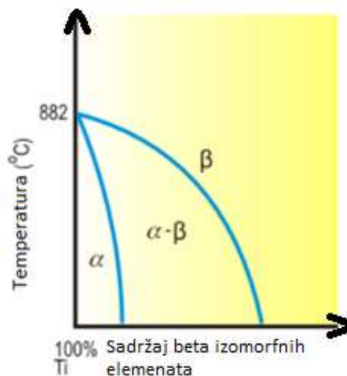
Slika 8. Utjecaj beta-izomorfni elemenata na titan [18]
