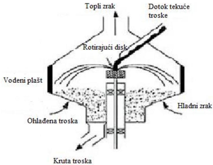
Slika 13. Atomizacija s rotirajućom „šalicom“ [28]
