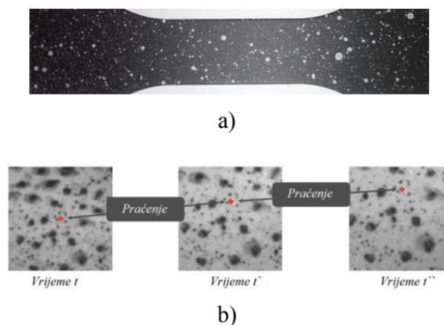
Slika 14. Uzorak za digitalnu korelaciju slike a) nasumično naneseeni markeri, b) praćenje pomaka markera [6]
