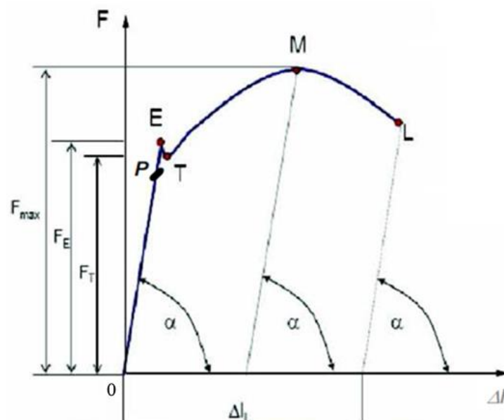
Slika 18. Dijagram sila ( F ) – produljenje ( \Delta l ) [23]
