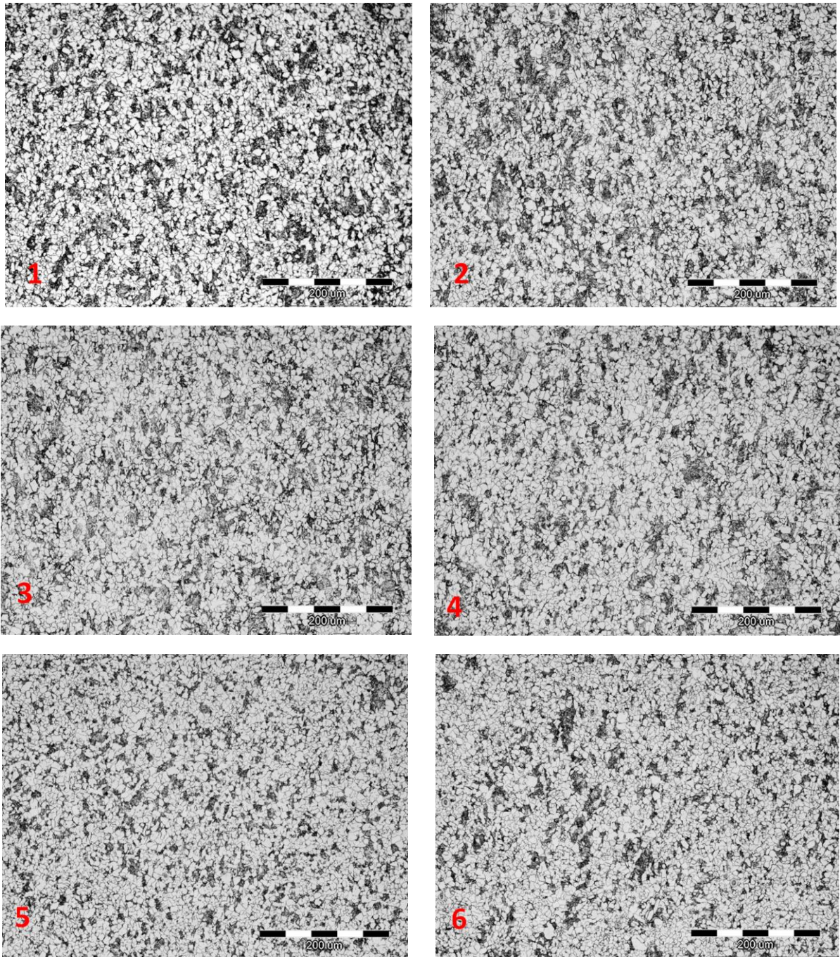
Slika 37. Mikrostruktura svake zone u trenutku zaustavljanja uzorka
