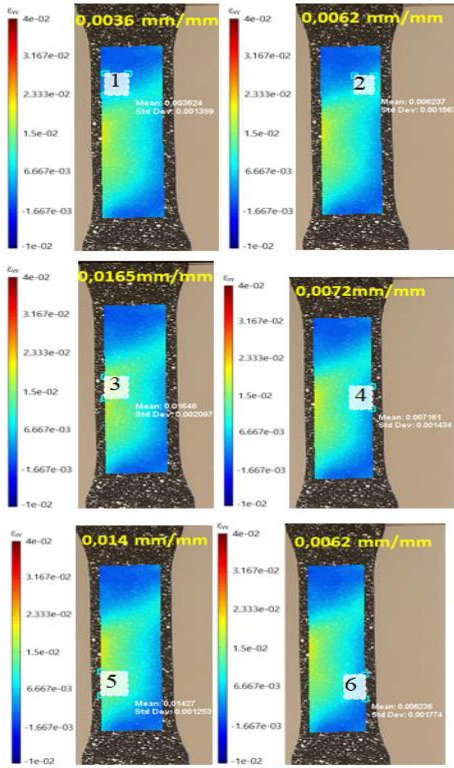
Slika 40. Iznos deformacije u svakoj zoni u trenutku zaustavljanja ispitivanja uzorka
