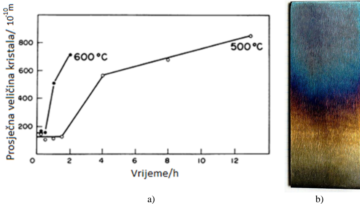
Slika 14. a) Prosječna veličina zrna NiO kao funkcija vremena [9] i b) interferencija svjetlosti na uzorku oksidiranoj čeliku [15]
